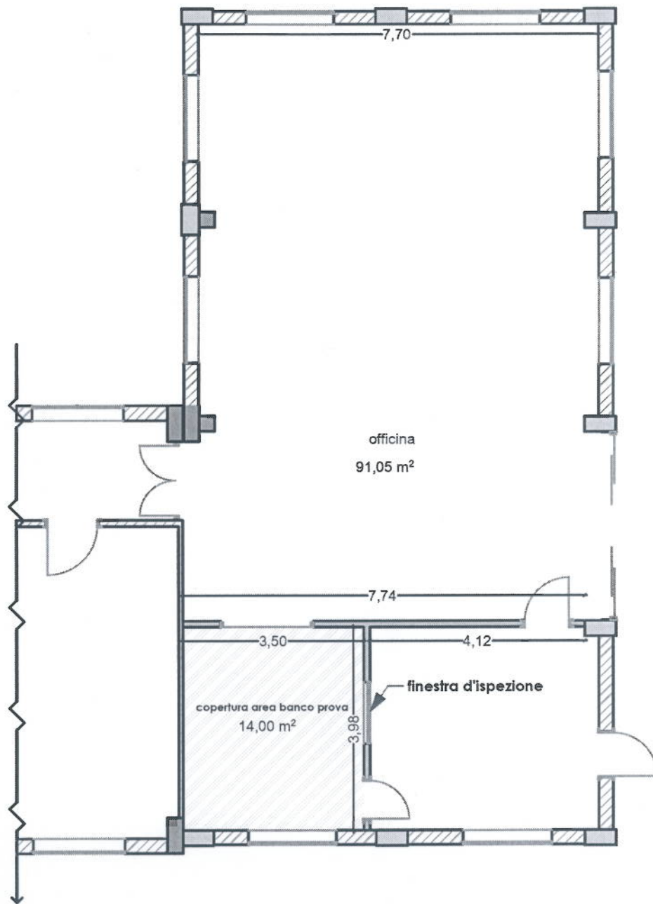
PLANIMETRIA SEDE MERCOGLIANO locale BANCO PROVA scala 1:100
